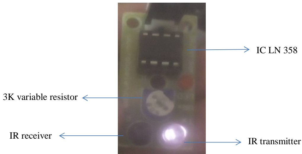
Fig 3. IR sensor module
